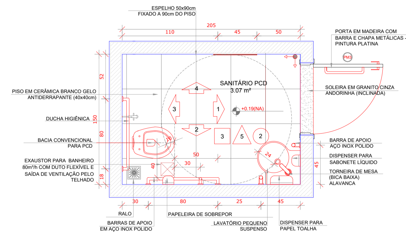
PLANTA BAIXA
