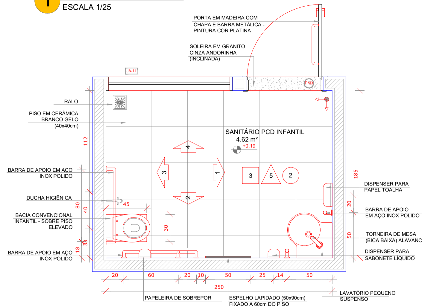
PLANTA BAIXA
